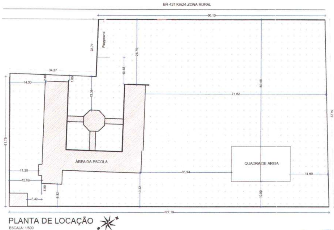
Figura 2: Planta de Locação da Escola Santa Lúcia. Em vermelho área edificada, em verde área livre.
